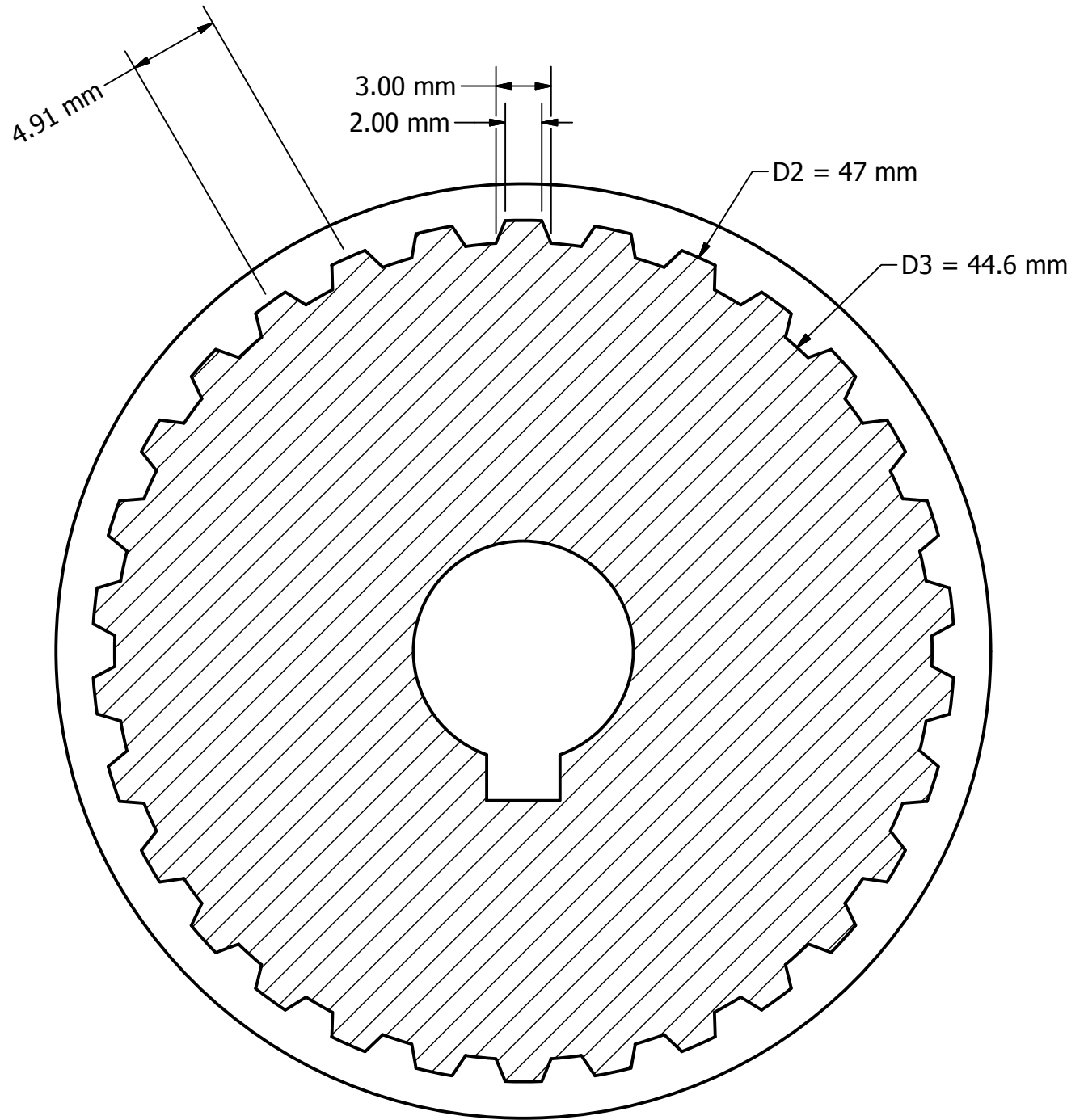
SECTION A-A SCALE 3 : 1
